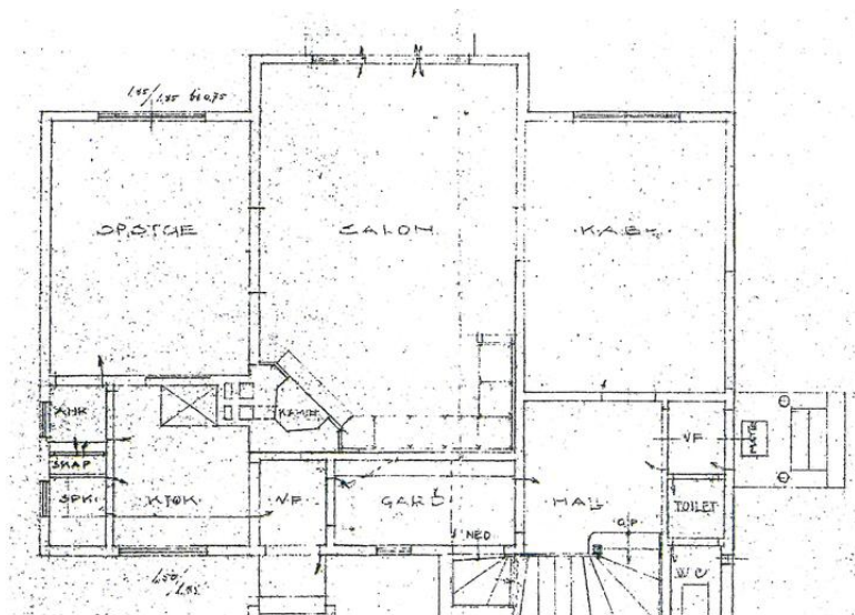
Plantegning av 1. etasje fra 1935. Opphavsrett: Statsbygg.
