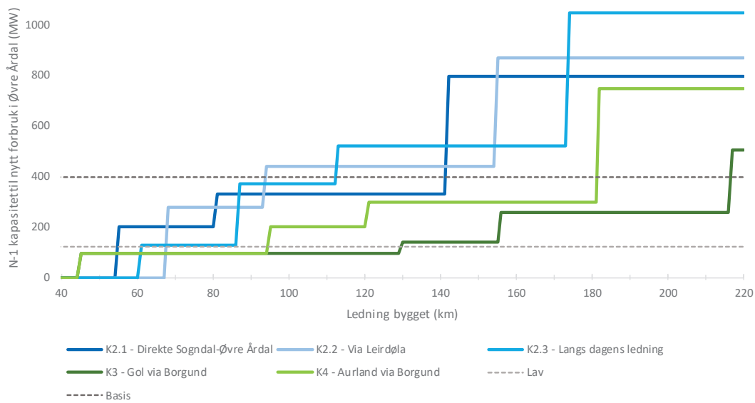
Figur 4-7 Kapasitetstrapp som viser hvordan N-1 kapasiteten til nytt forbruk i Øvre Årdal utvikler seg i hvert byggetrinn i de ulike konseptene, forutsatt at vi har gjennomført mindre tiltak. Figuren inkluderer reinvestering av dagens 300 kV-ledning Sogndal-Leirdøla-Jamnene og tilhørende spenningsheving til 420 kV.
