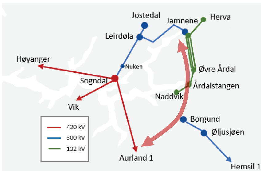
Figur 4-5 Illustrasjon av konsept 4 – ny ledning mot Borgund og videre mot Aurland.
