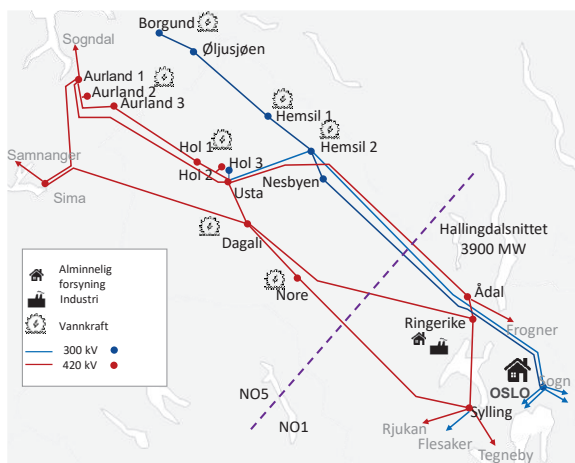
Figur 2-2 Transmisjonsnett i Hallingdal slik det ser ut i dag. Stiplet linje indikerer Hallingdalsnettet.
