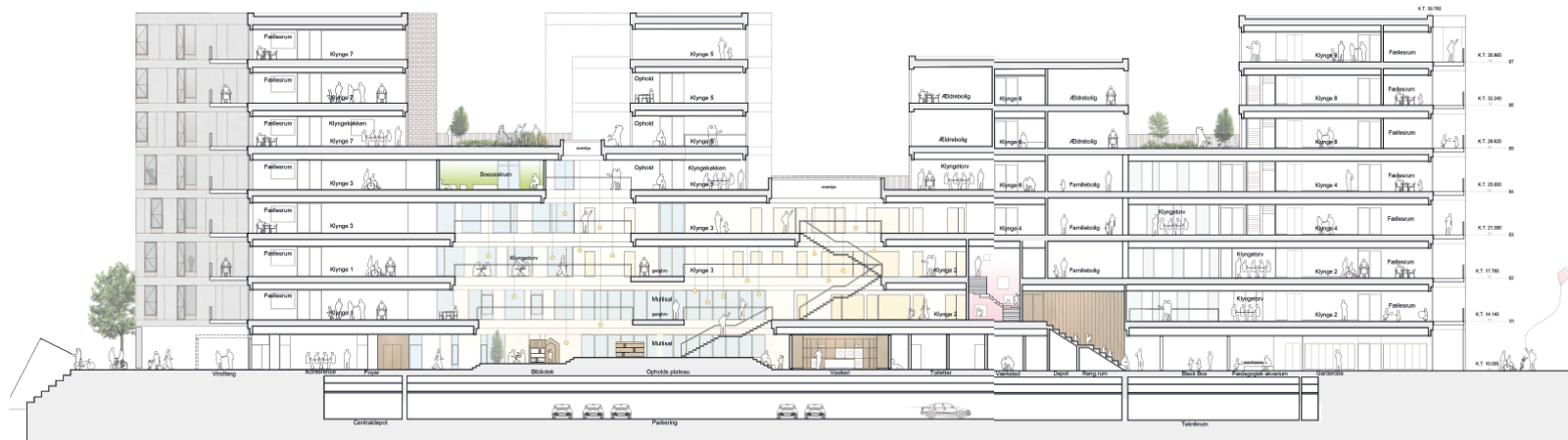
Længdesnit 1:200
