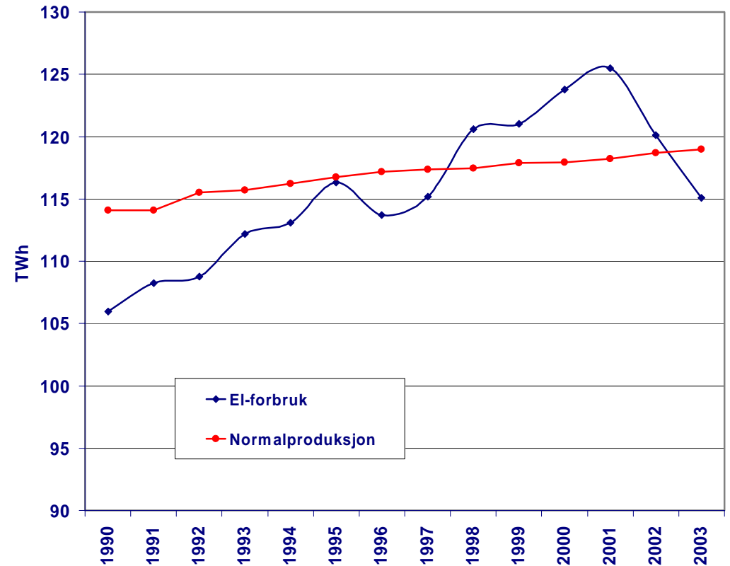
Utviklingen i produksjonskapasitet og kraftforbruk
